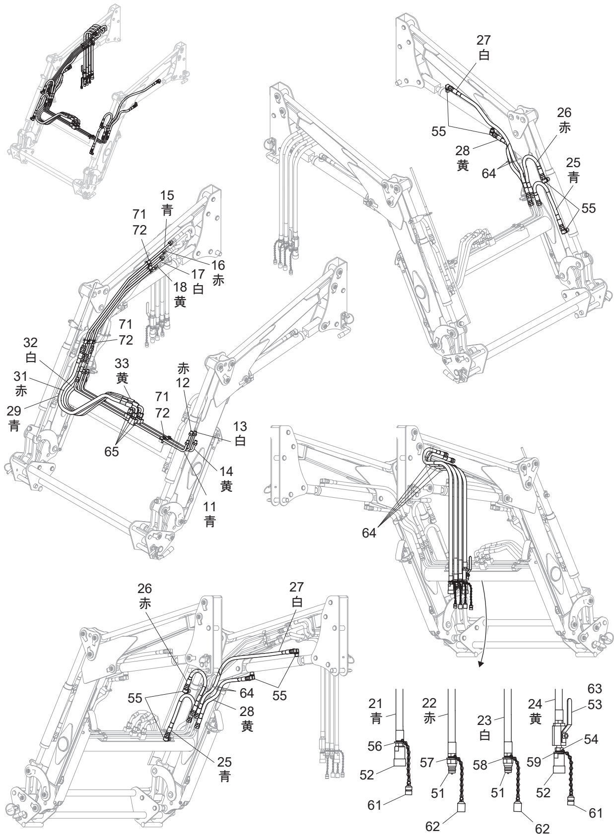
Fig. 2 パイピング
