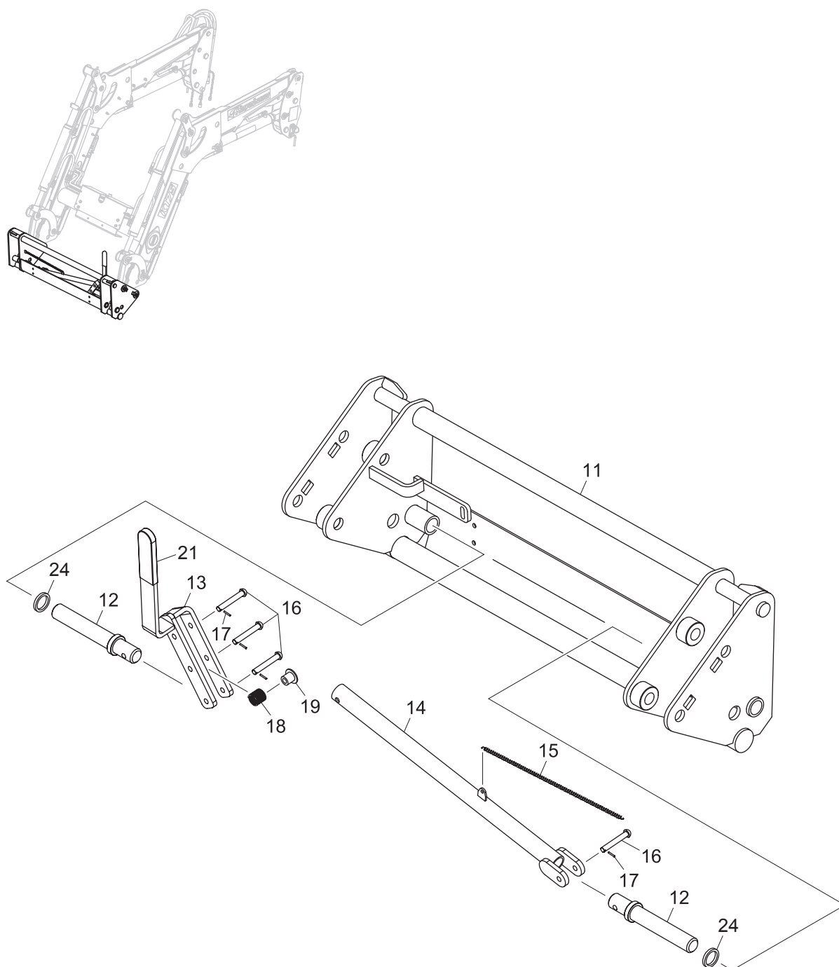
Fig. 8 バケットヒッチ (レバー式)
