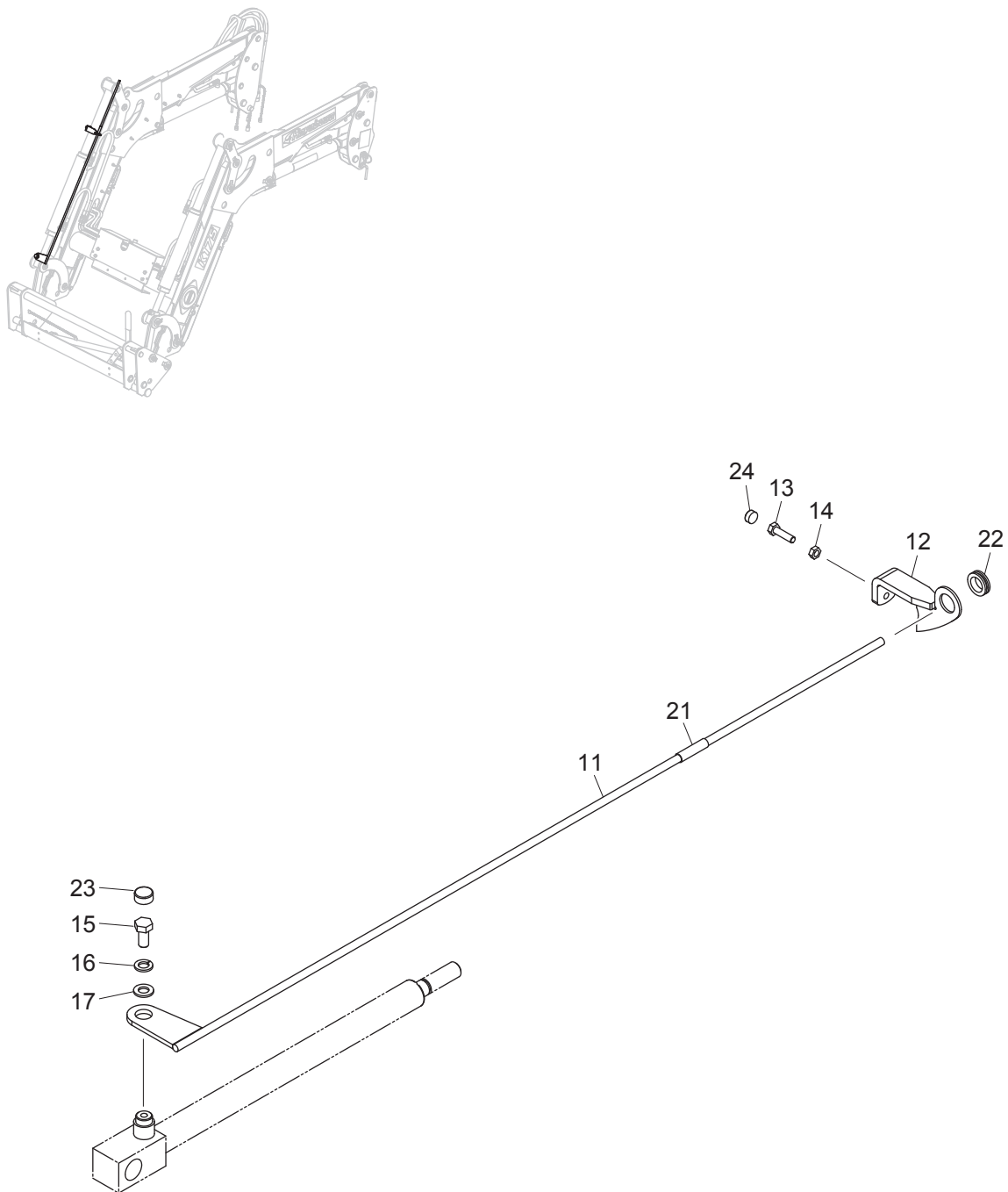
Fig. 7 レベラー
