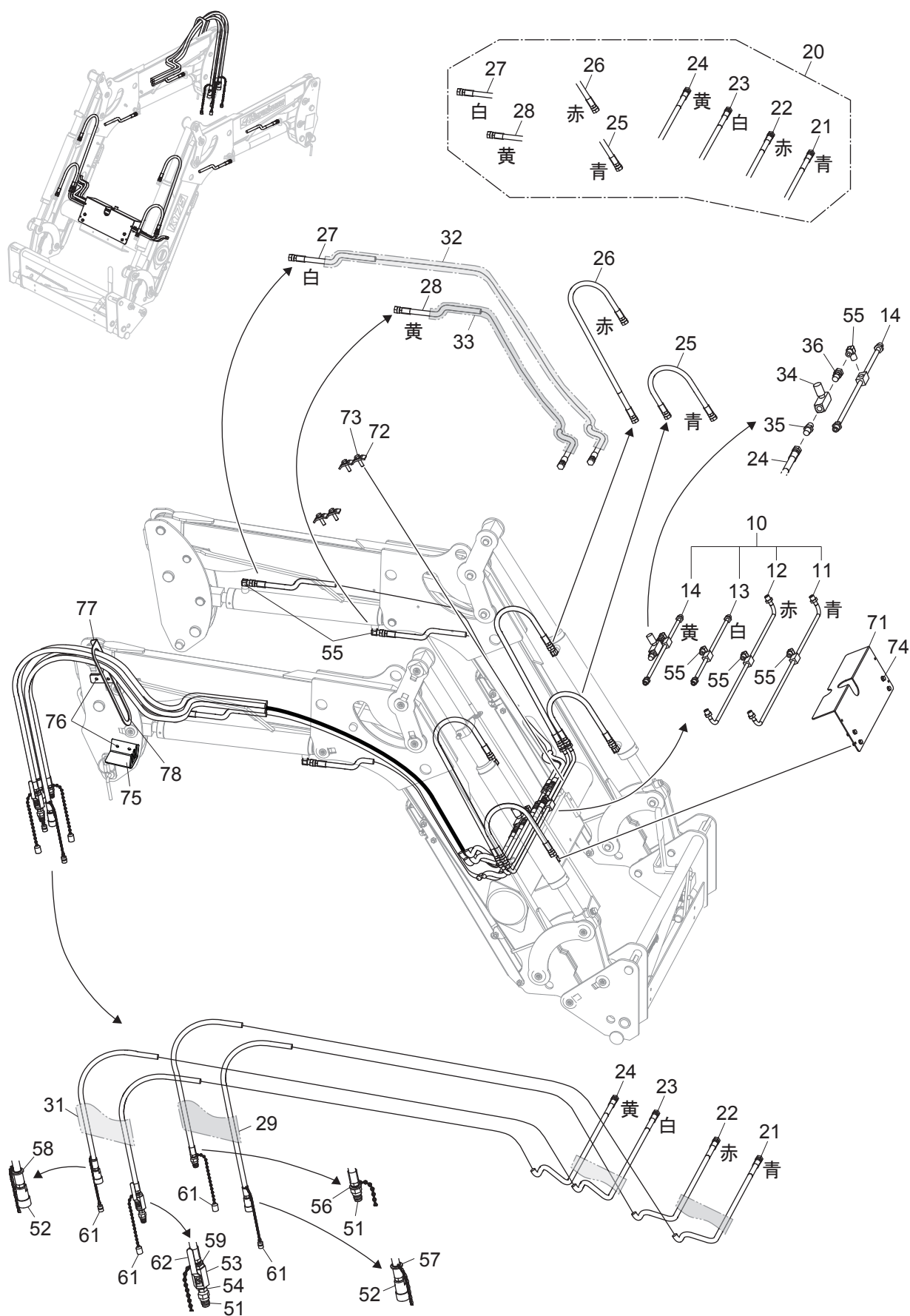
Fig. 2 パイピング
